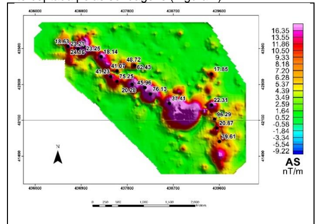
Figura 2: ASA com as soluções de Euler. Os números indicam a profundidade das fontes..
