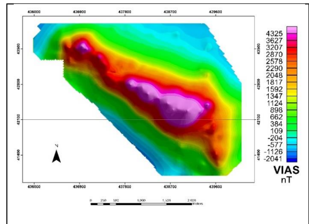
Figura 5: Mapa do VIAS para o depósito do Pelado.
